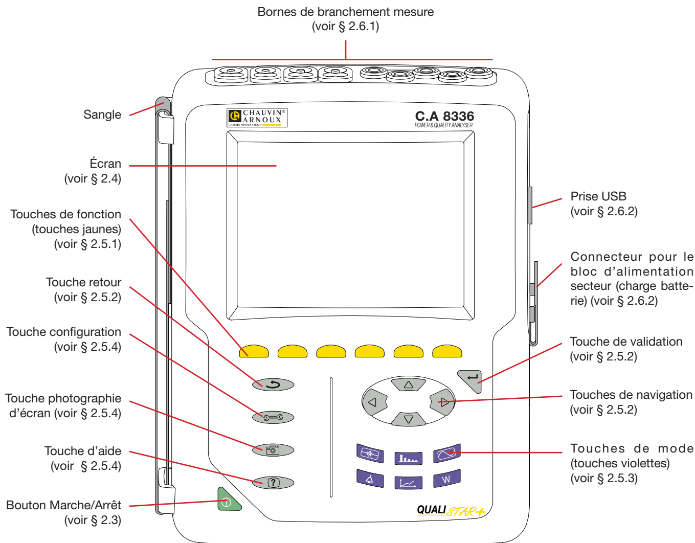
Figure 1 : vue générale du Qualistar+
