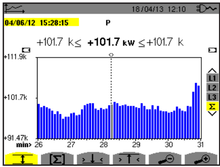
Figure 100 : P (Σ) avec MIN-AVG-MAX
