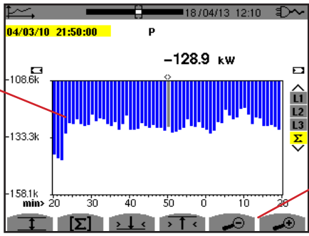
Figure 99 : P (Σ) sans MIN-AVG-MAX
