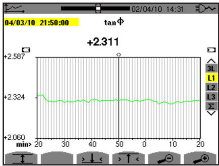
Figure 97 : tan Φ (L1) sans MIN-AVG-MAX pour un branchement triphasé avec neutre
