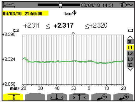
Figure 98 : tan Φ (L1) avec MIN-AVG-MAX
