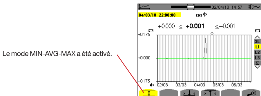
Figure 104 : cos \Phi (L1) avec MIN-AVG-MAX
